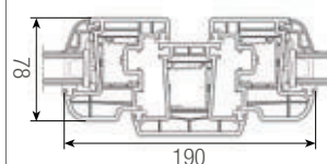
słupek 86 – skrzydło 60
