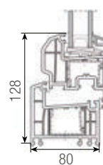
ościeżnica 68 – skrzydło A 60
