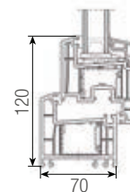
ościeżnica 68 – skrzydło Z 60
