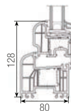
ościeżnica 76-80 – skrzydło 60
